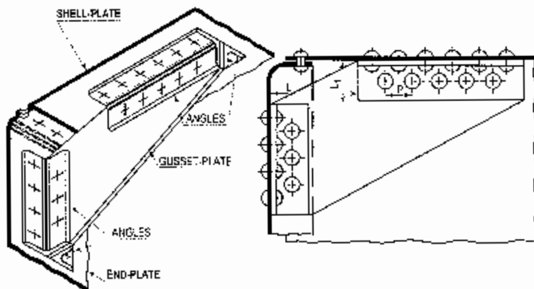
Gussier stay (Fig. 25-11)
